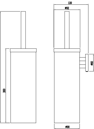
WSPAPTBCP/BN/GM WSELTBH
