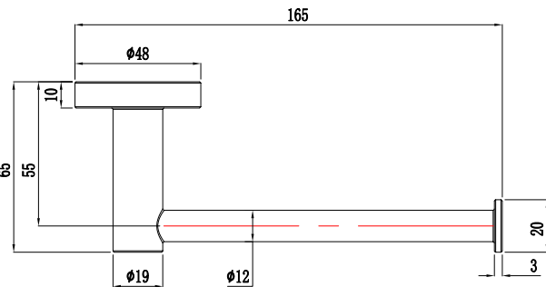
WSPAPTBCP/BN/GM WSELTBH
