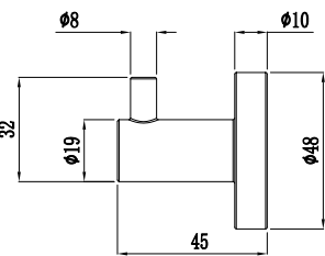
WSPINRHCP/BN/GM WSEMHHMB
