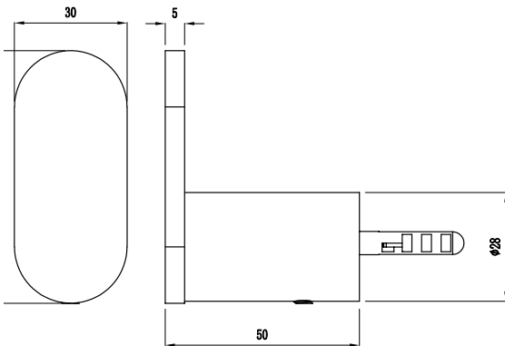
WSPRHCP/WSELRHMB WSPAPRHBN/GM
